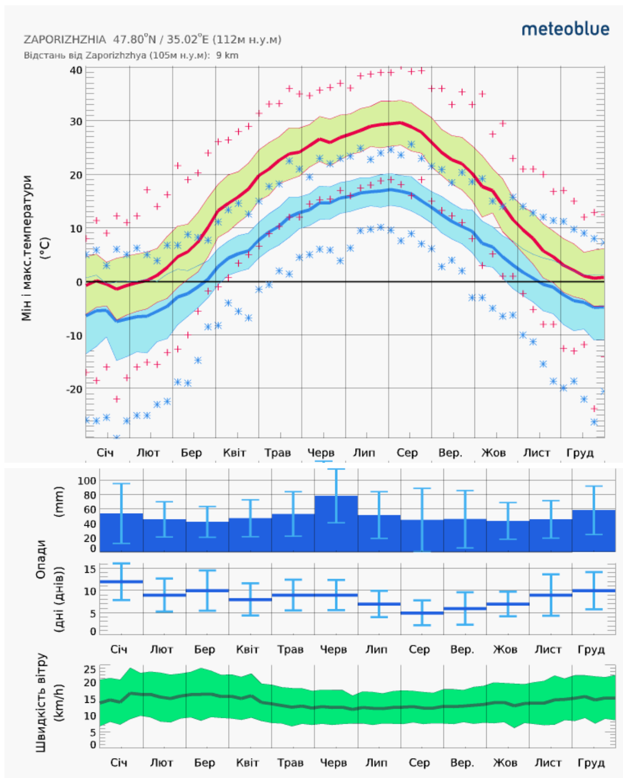
Рис.2.7. Розподіл основних метеопказників по станції Запоріжжя [4] .
