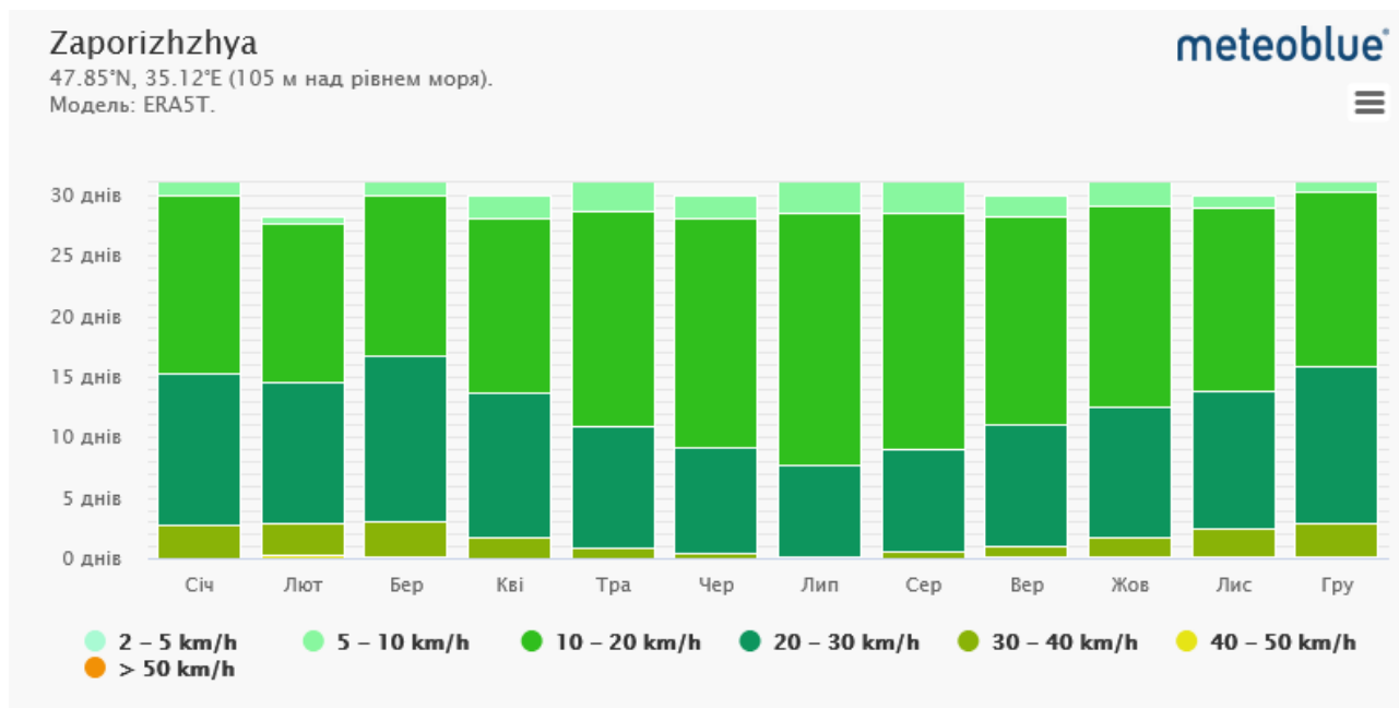
Рис.2.5. Швидкість вітру [4] .
